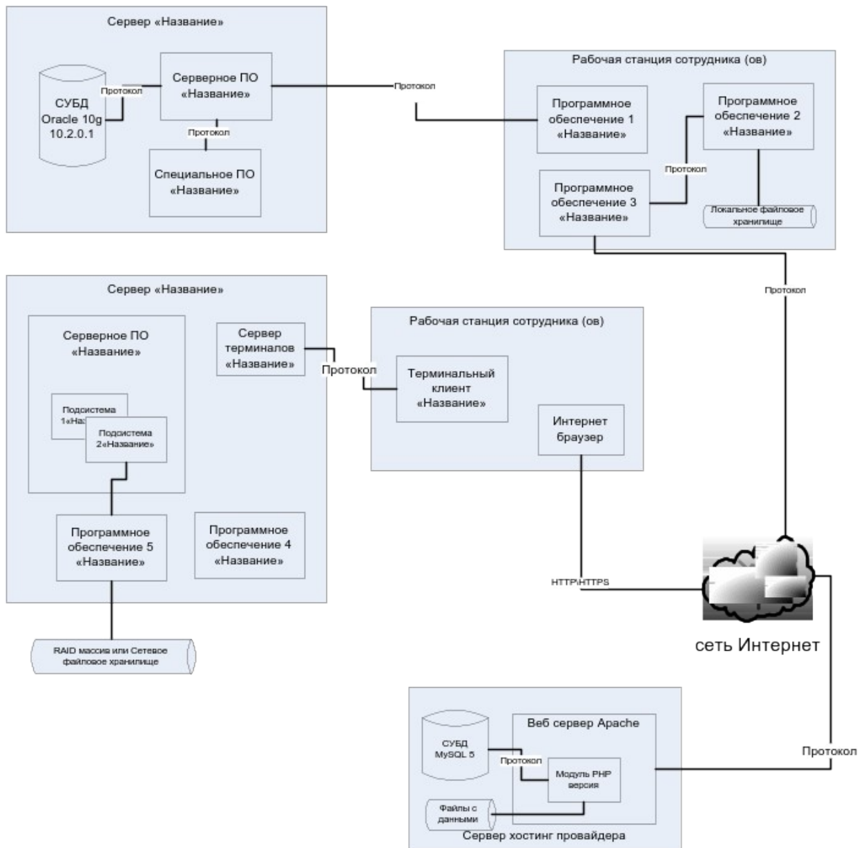
Общий пример представления программной архитектуры
